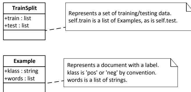
Gambar 8 Dua buah inner class dari kelas Naïve Bayes
